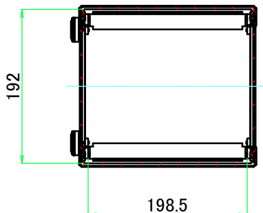
B-B ( 1 : 6.5 )
