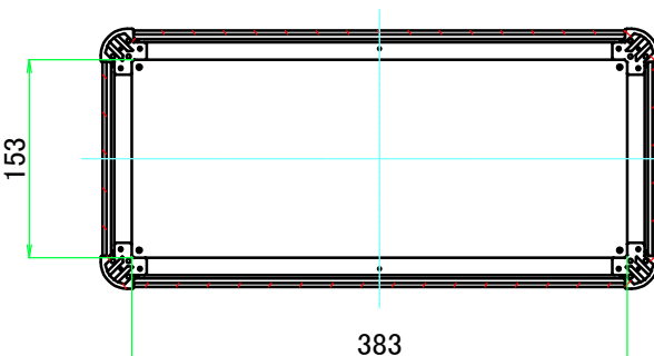
C-C ( 1 : 6.5 )
